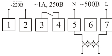
Рис. 9 – Схема подключения прибора. Тип корпуса P77
