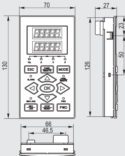
Панель управления AFD-XPNL.21 используется с ПЧ AFD-E055.43В и выше
