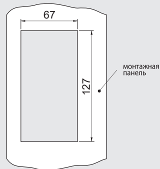
панели AFD-XPNL.21 и AFD-XPNL.22
