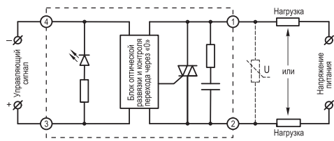
Схема твердотельного реле со встроенной RC-цепью
