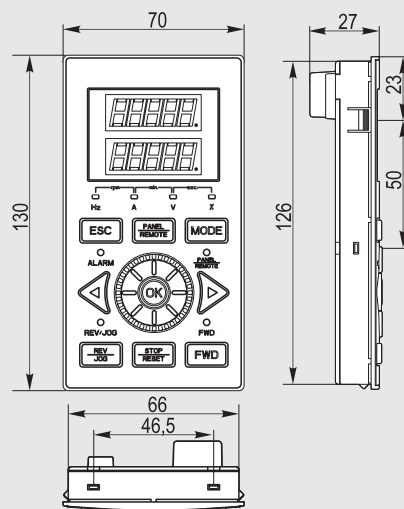
Панель управления AFD-XPNL.22 Используется с ПЧ AFD-E055.43В и выше
