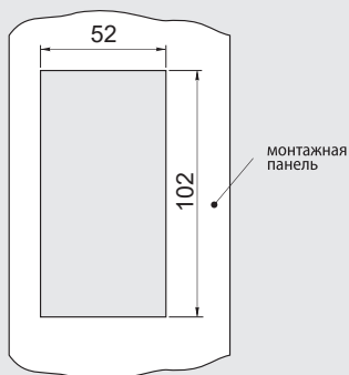
панели AFD-XPNL.11 и AFD-XPNL.12
