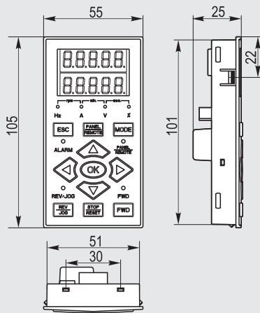
Панель управления AFD-XPNL.21 используется с ПЧ AFD-E055.43В и выше
